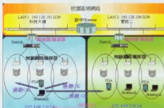
東海大學校園無線區域網路架構圖。
