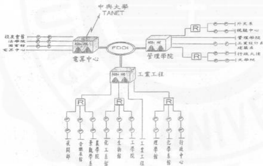
東海大學第一期校園FDDI光纖網路系統圖
